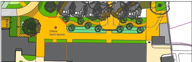
Plan et Coupe de l'agrandissement du boisement par la réduction de la voirie côté Nord du bâtiment Habitation
