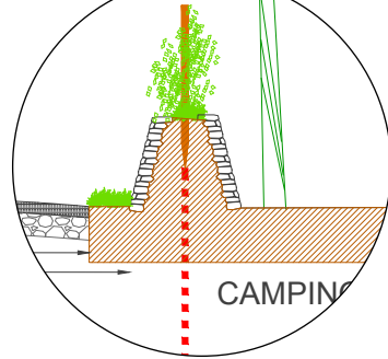
Coupe des Talus à créer
